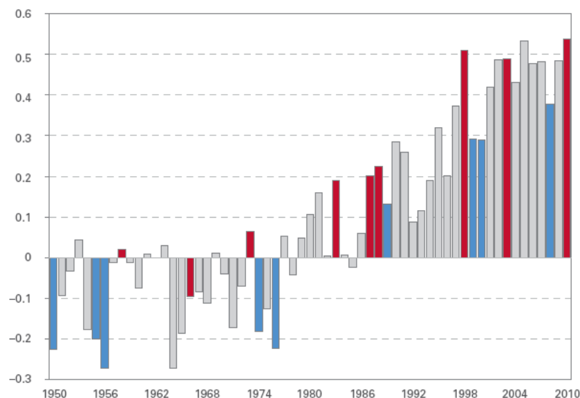
Slika 6.1.1-2 Anomalije globalne površinske temperature (°C) za razdoblje 1950-2010. godine u odnosu na standardno razdoblje 1961.-1990. godine uz označavanje godina s pojavom La Nina (plavo) i El Nino (crveno). (WMO, 2013.)
