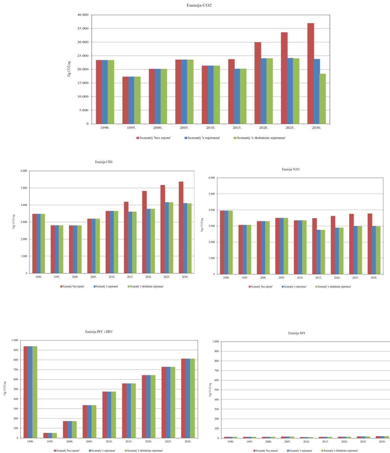
Slika 5.3-1: Projekcije emisija stakleničkih plinova po plinovima
