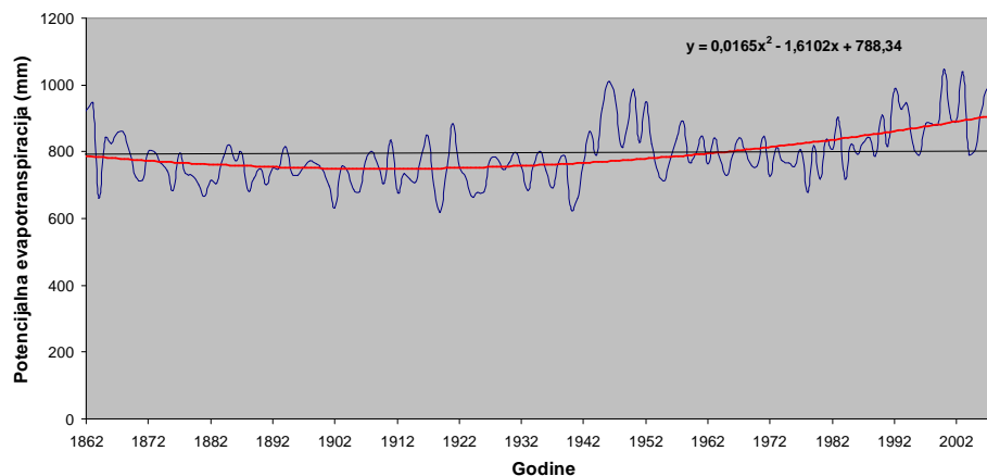
Slika 6.2.4-1. Godišnja potencijalna evapotranspiracija (u milimetrima) za meteorološku postaju Zagreb-Grič za razdoblje 1862.-2008. godine. Tanka crta predstavlja prosjek za razdoblje 1961.-1990. godina (Pandžić i Trninić, 2010)
