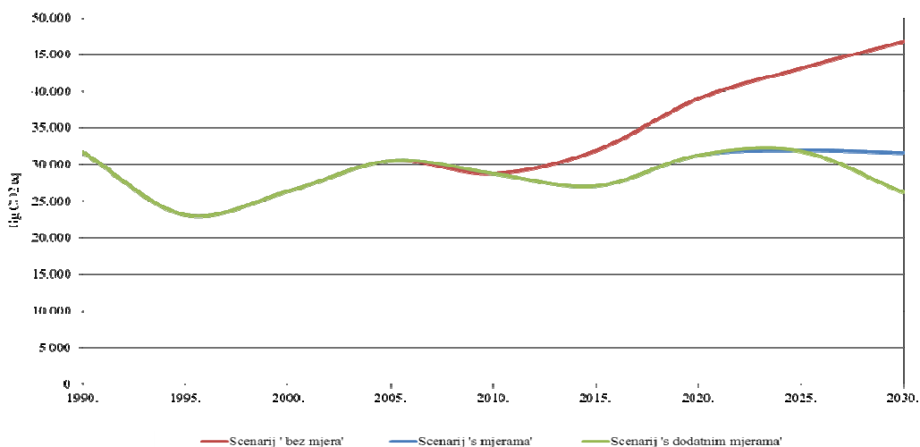
Slika 5.4-1: Povijesne emisije i ukupne projekcije emisija stakleničkih plinova
