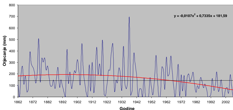
Slika 6.2.4-2 Izračunata godišnja otjecanja (u milimetrima) za meteorološku postaju Zagreb-Grič za razdoblje 1862.-2008. godina. Tanka crta predstavlja prosjek za razdoblje 1961.-1990.godine (Pandžić i Trninić, 2010)
