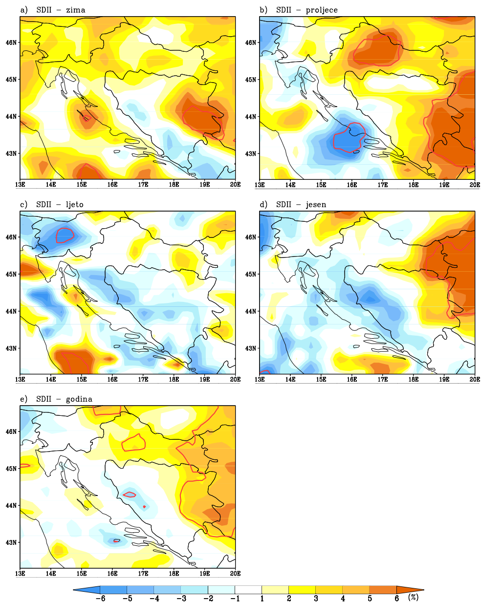
Slika 6.3.3.2-3. Promjena dnevnog intenziteta oborine (SDII) po sezonama (a-d) i za godinu (e) u bližoj budućnosti (2011.-2040. godina, P1) u odnosu na referentno razdoblje (1961.-1990. godina, P0). Promjene su izražene u postocima intenziteta u referentnom razdoblju. Statistički značajne promjene na 95% razini povjerenja su označene crvenom krivuljom
