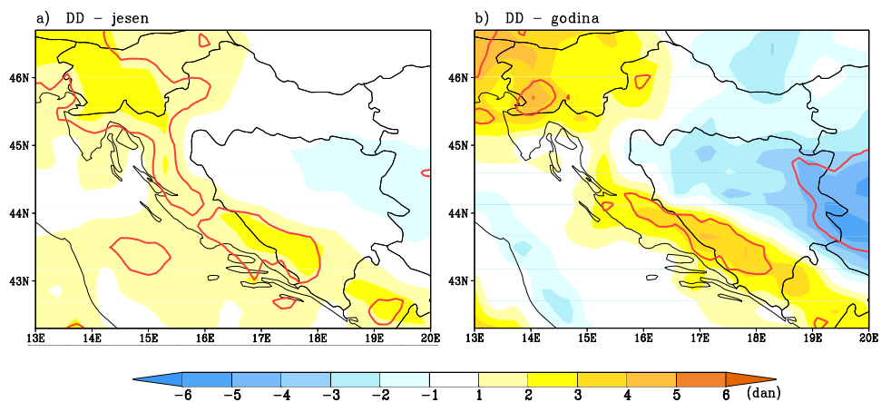
Slika 6.3.3.2-2. Promjena broja suhih dana (DD) u bližoj budućnosti (2011.-2040. godina) u odnosu na referentno razdoblje (1961.-1990. godina) u jesen (a) i za godinu (b). Statistički značajne promjene na 95% razini povjerenja su označene crvenom krivuljom
