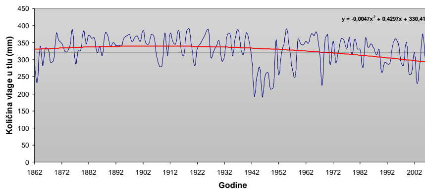
Slika 6.2.4-3. Izračunate godišnje količine vlage u tlu (u milimetrima) za meteorološku postaju Zagreb-Grič za razdoblje 1862.-2008. godine. Tanka linija predstavlja prosjek za razdoblje 1961.-1990. godine (Pandžić i Trninić, 2010).
