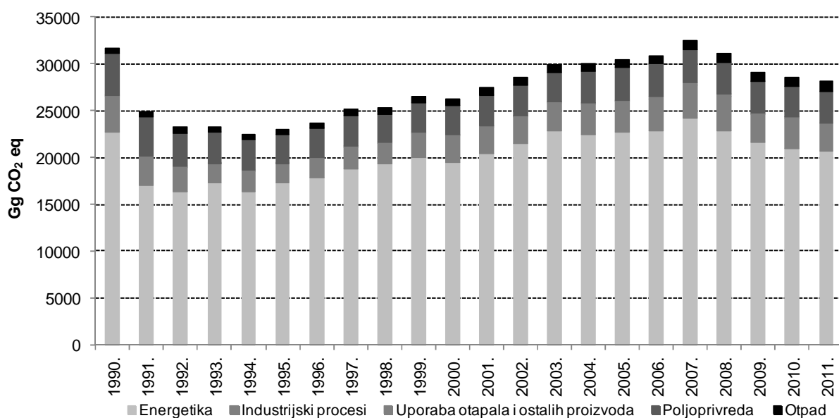
Slika 3.2-2: Trend emisija stakleničkih plinova, po sektorima
