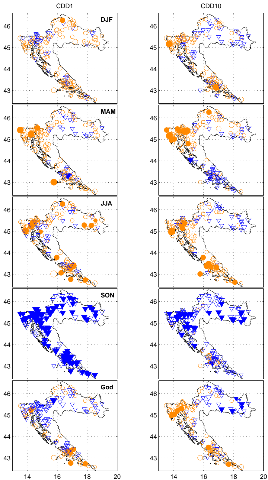
Slika 6.2.3-1. Dekadni trendovi (%/10god) maksimalnih sušnih razdoblja za kategorije 1mm i 10 mm (CDD1, CDD10), po sezonama i za godinu u razdoblju 1961.-2010. godine. Krugovi označavaju pozitivne trendove, trokuti negativne, dok popunjeni znakovi označavaju statistički značajan trend. Četiri veličine znakova su proporcionalne relativnim vrijednostima promjena na desetljeće u odnosu na odgovarajući srednjak iz razdoblja 1961.-1990. godine: <5%, 5-10%, 10-30% i >30%
