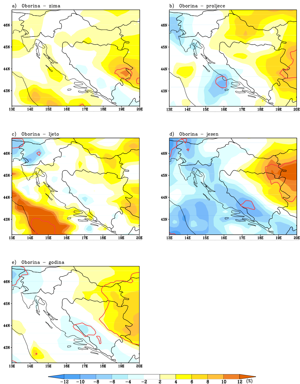
Slika 6.3.3.2-1. Promjena sezonske (a-d) i godišnje količine oborine (e) u bližoj budućnosti (2011.-2040. godina, razdoblje P1) u odnosu na referentno razdoblje (1961.-1990. godina, P0). Promjene su izražene u postocima količina oborine u referentnom razdoblju. Statistički značajne promjene na 95% razini povjerenja označene su crvenom krivuljom
