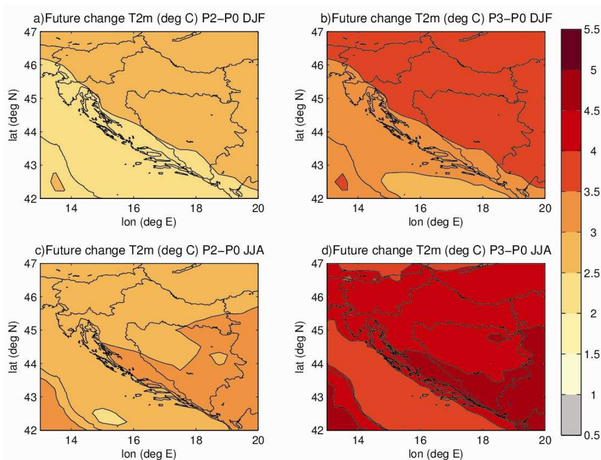
Slika 6.3.3.1-5. Razlika srednjaka skupa u T2m: zima (DJF) a) P2-P0 i b) P3-P0 te ljeto (JJA) c) P2-P0 i d) P3-P0. Mjerene jedinice su °C. U svim točkama dvije trećine modela daje isti predznak promjene kao srednjak skupa svih modela
