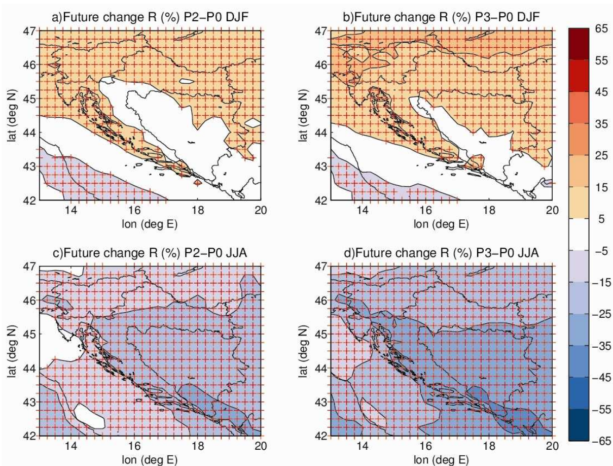
Slika 6.3.3.2-7. Relativna razlika srednjaka skupa za ukupnu količinu oborine R : klimatološka zima (DJF) a) P2-P0 i b) P3-P0 te ljeto (JJA) c) P2-P0 i d) P3-P0. Mjerene jedinice su %. S oznakom + su označene točke u kojima dvije trećine modela daje isti predznak promjene kao srednjak skupa te je relativna razlika srednjaka skupa izvan intervala \pm 5\% .
