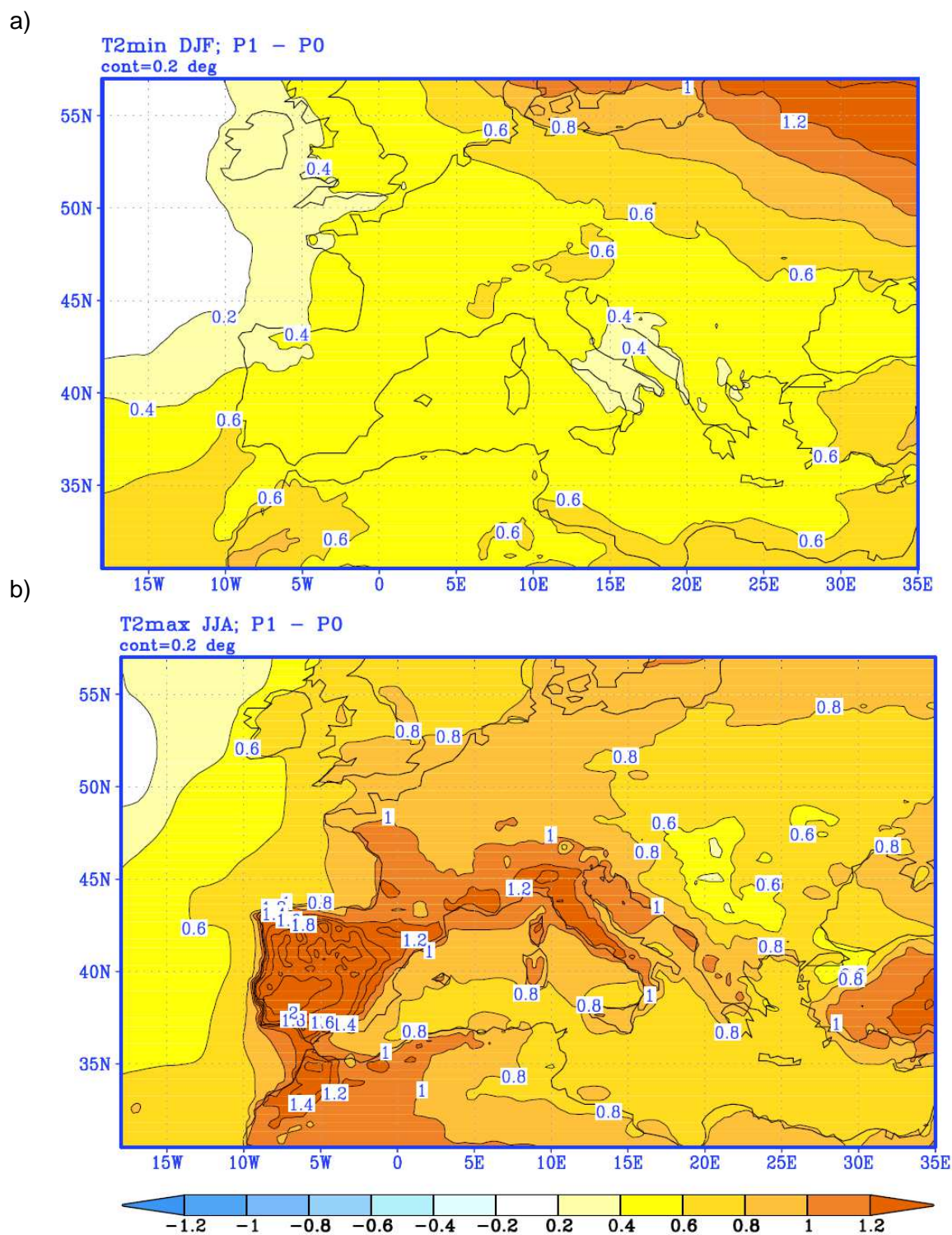
Slika. 6.3.3.1-2. Srednjak ansambla a) minimalne T2m zimi i b) maksimalne T2m ljeti, P1 minus P0. Izolinije svaka 0,2 °C
