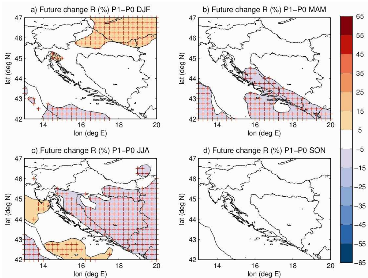
Slika 6.3.3.2-6. Relativna razlika srednjaka skupa za ukupnu količinu oborine R između razdoblja P1 i P0 : a) zima (DJF), b) proljeće (MAM), c) ljeto (JJA) i d) jesen (SON). Mjerene jedinice su %. S oznakom + su označene točke u kojima dvije trećine modela daje isti predznak promjene kao srednjak skupa svih modela te je relativna razlika srednjaka skupa izvan intervala \pm 5\%
