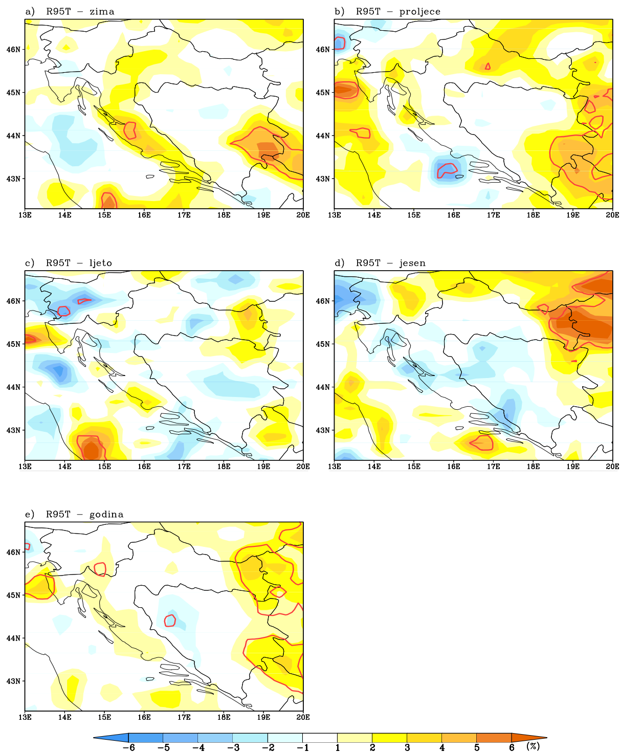
Slika 6.3.3.2-5. Promjena udjela sezonske (a-d) i godišnje (e) količine oborine koja padne u vrlo vlažne dane u ukupnoj sezonskoj odnosno godišnjoj količini oborine (R95T) u bližoj budućnosti (2011.-2040.; P1) u odnosu na referentno razdoblje (1961.-1990.; P0). Promjene su izražene kao razlike vrijednosti indeksa u budućoj i sadašnjoj klimi. Statistički značajne promjene na 95% razini povjerenja su označene crvenom krivuljom
