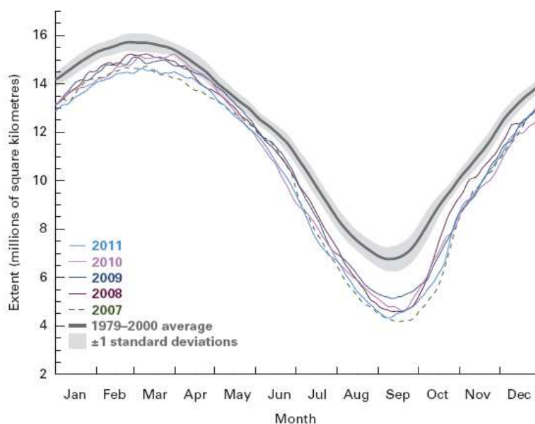
Slika 6.1.3-1 Ledeni morski pokrov sjeverne hemisfere za 2011. godinu u usporedbi s prethodnim godinama i prosjekom za razdoblje 1979.-2000. godine
