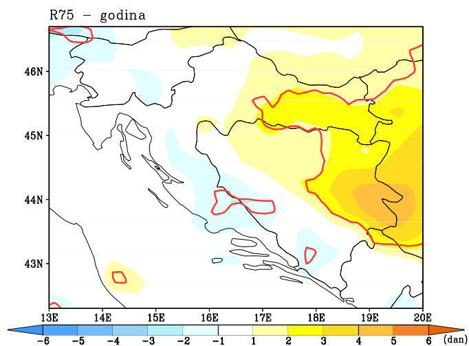
Slika 6.3.3.2-4. Promjena vlažnih dana (R75) u godini u bližoj budućnosti (2011.-2040. godina, P1) u odnosu na referentno razdoblje (1961.-1990. godina, P0). Promjene su izražene kao razlike vrijednosti indeksa u budućoj i sadašnjoj klimi. Statistički značajne promjene na 95% razini povjerenja su označene crvenom krivuljom.
