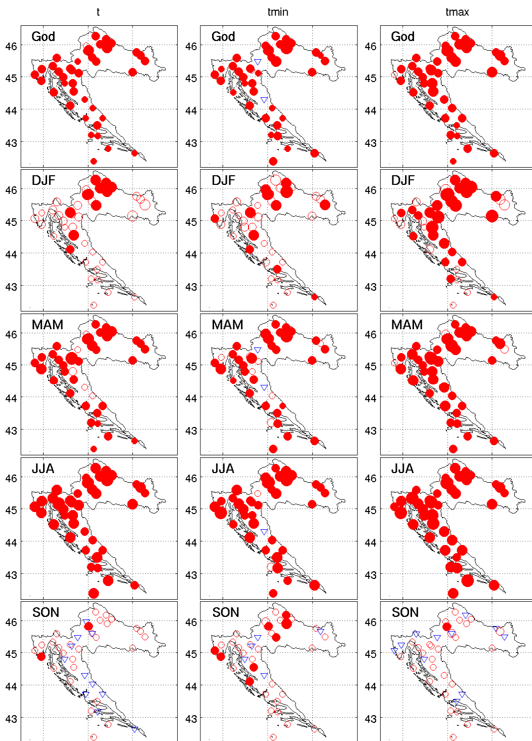
Slika 6.2.1-1. Dekadni trendovi ( ^{\circ}\text{C}/10\text{god} ) srednje ( t ), srednje minimalne ( t_{\text{min}} ) i srednje maksimalne ( t_{\text{max}} ) temperature zraka za godinu i po godišnjim dobima (DJF – zima, MAM – proljeće, JJA – ljeto, SON – jesen) u razdoblju 1961.-2010. godine. Krugovi označavaju pozitivne trendove, trokuti negativne, dok popunjeni znakovi označavaju statistički značajan trend. Četiri veličine znakova su proporcionalne promjeni temperature u ^{\circ}\text{C} na desetljeće.
